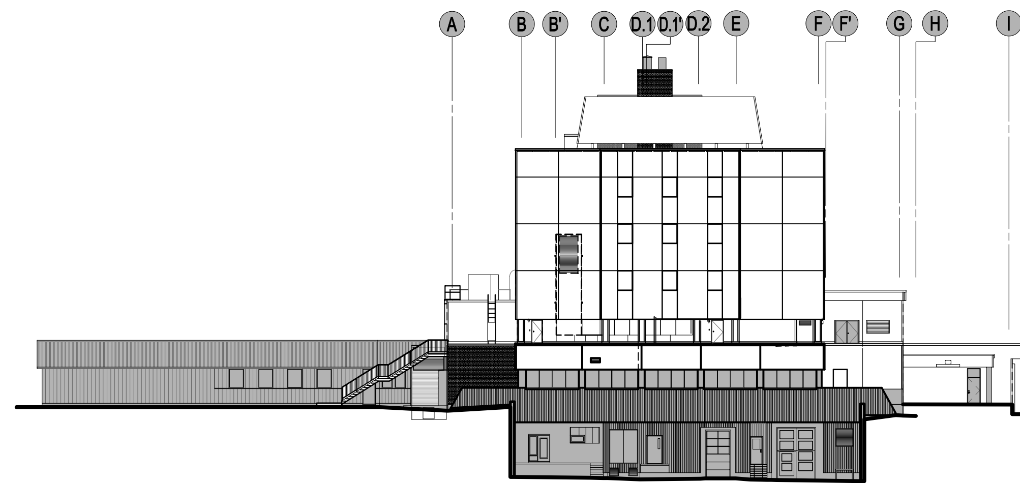
B ÉLÉVATION OUEST 1:300mm
