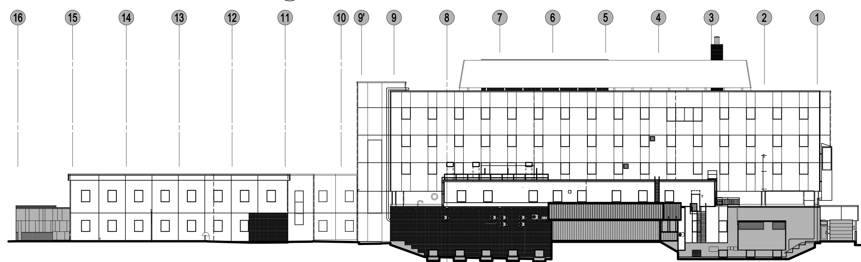
B ÉLÉVATION OUEST 1:300mm
