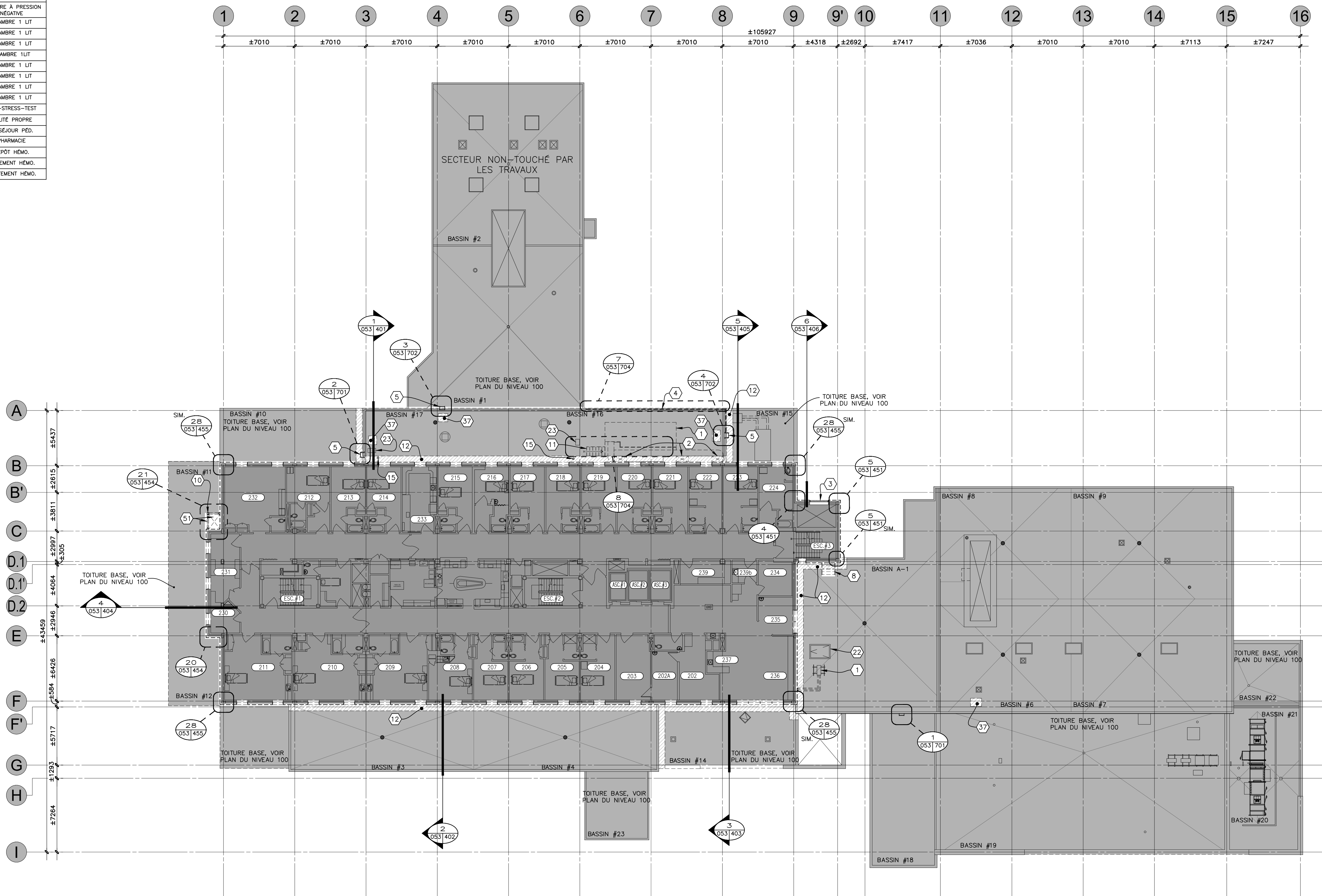
PLAN DU NIVEAU 200 - DÉMOLITION
